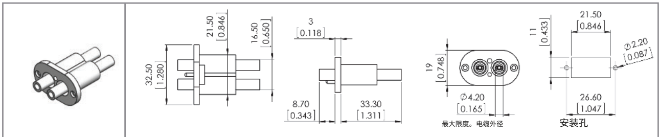
图纸 - 尺寸, 单位为毫米 [英寸]
