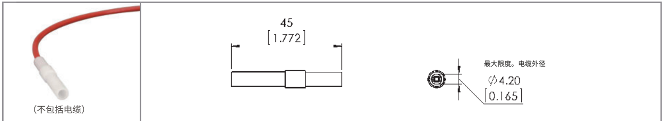
图纸 - 尺寸, 单位为毫米 [英寸]
