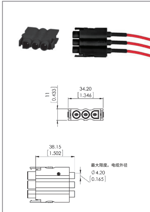
图纸 - 尺寸, 单位为毫米 [英寸]
