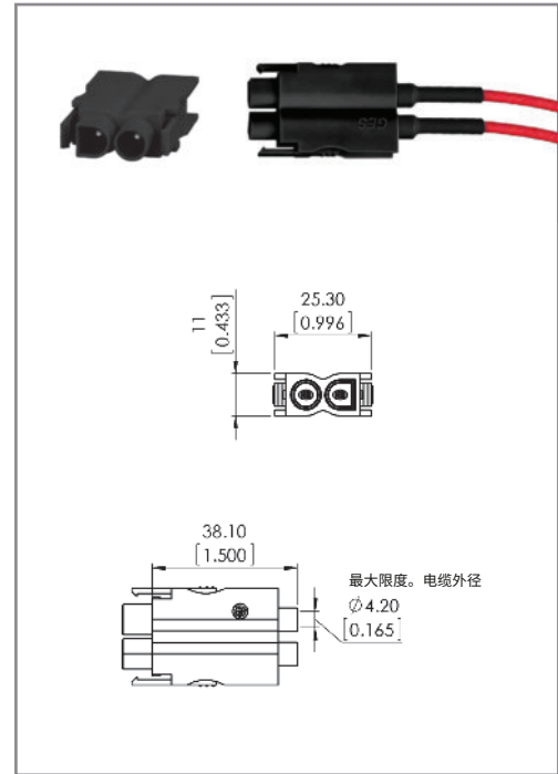
图纸 - 尺寸, 单位为毫米 [英寸]
