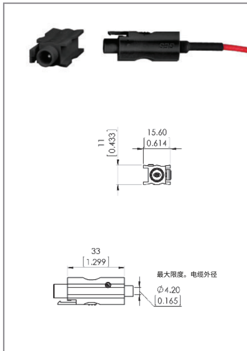
图纸 - 尺寸, 单位为毫米 [英寸]
