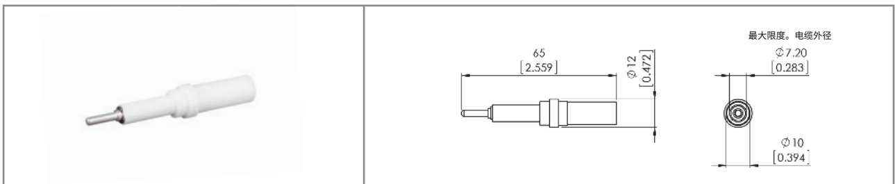
图纸 - 尺寸, 单位为毫米 [英寸]
